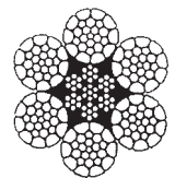
6 x WS(26)IWRC
